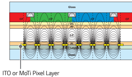
ITO or MoTi Pixel Layer
